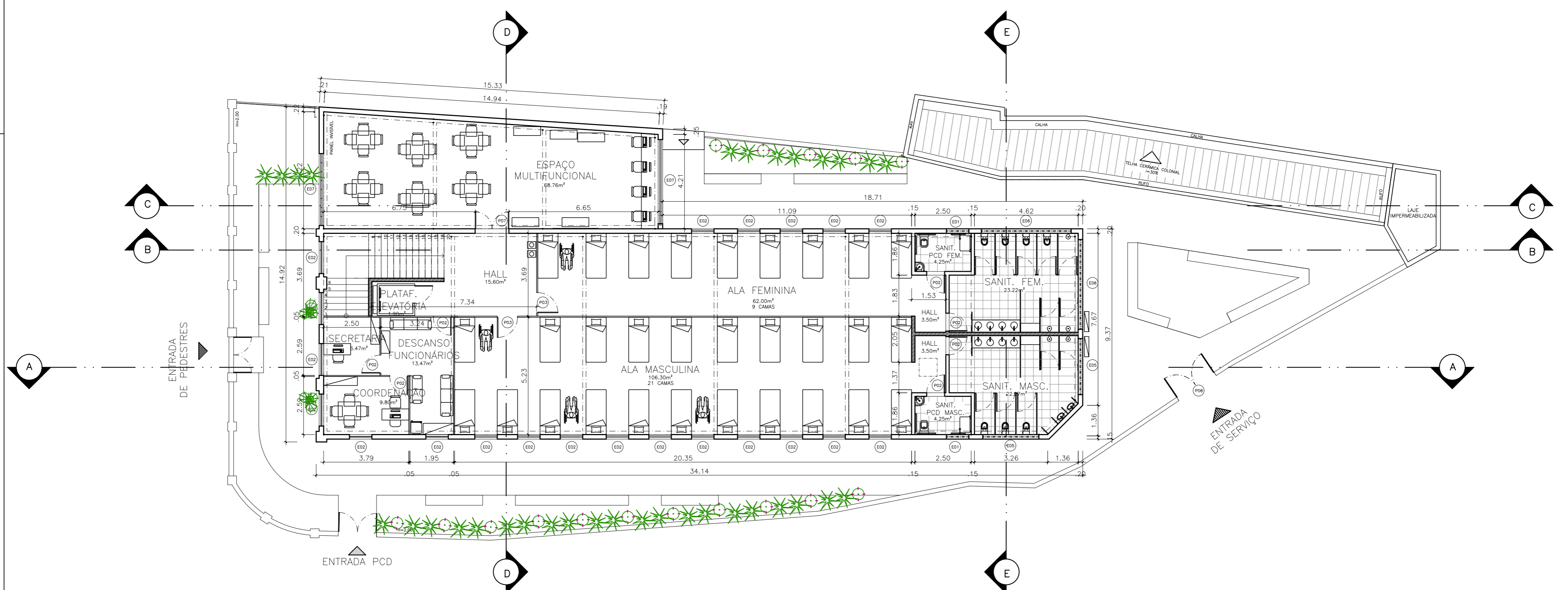
PLANTA BAIXA PAVIMENTO SUPERIOR
